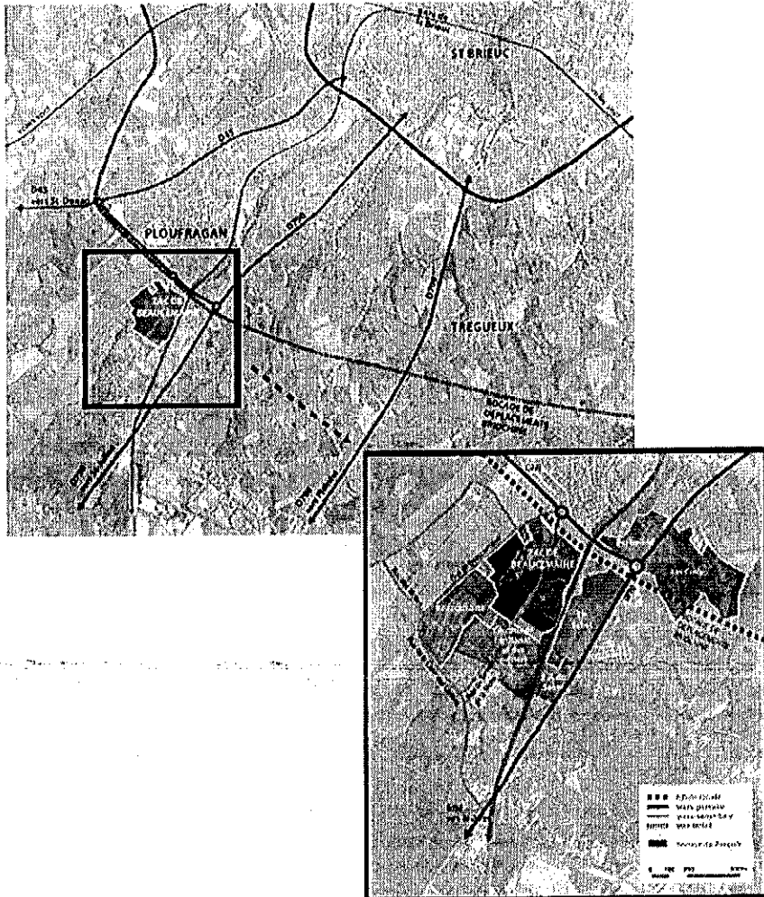
Plan de situation de la ZAC de Beaucemaine, extrait du dossier de création
